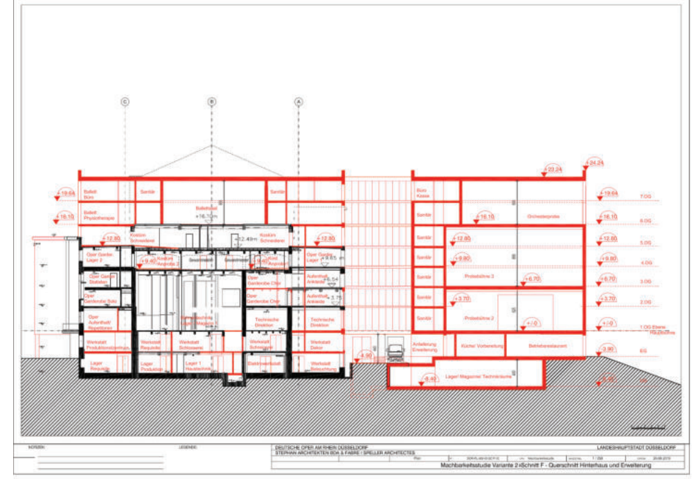
Schnitt FF
