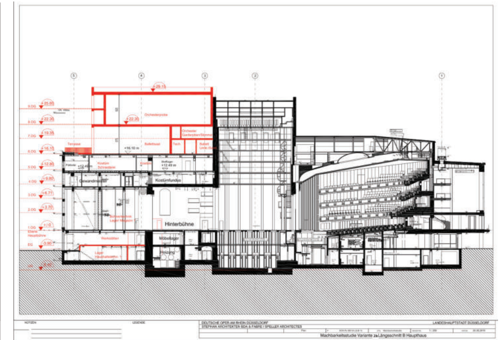
Schnitt BB
