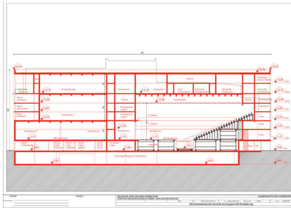
Schnitt GG
