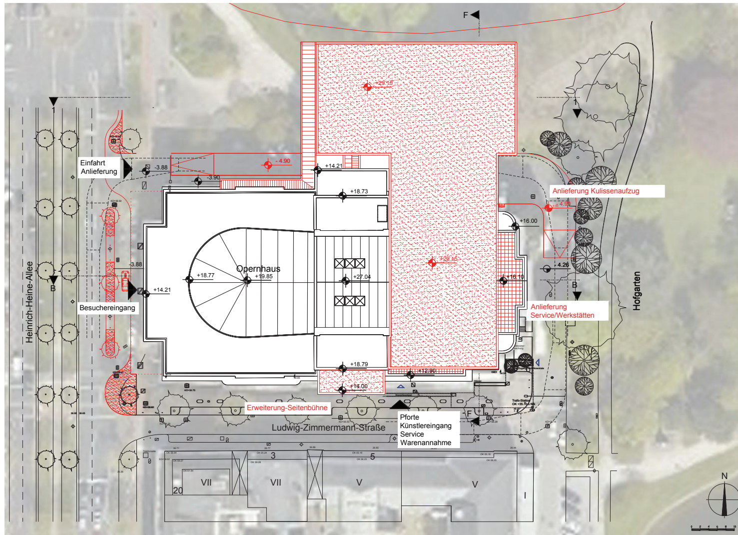
Lageplan
